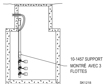
SUPPORT DE FLOTTES TYPIQUE POUR PUISSARD EN BÉTON OU POUR PUIT D'ACCÈS DE FOSSE SEPTIQUE
