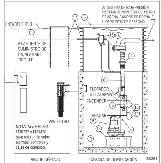
INSTALACIÓN TÍPICA PARA EFLUENTES
