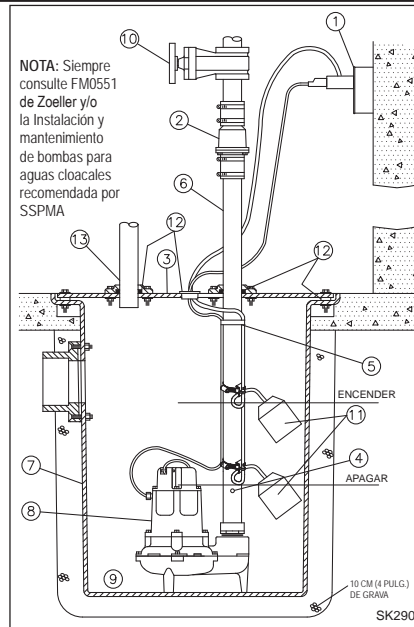
INSTALACIÓN TÍPICA PARA AGUAS CLOACALES
