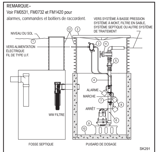
INSTALLATION TYPIQUE POUR LES EFFLUENTS
