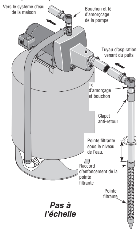
Figure 1: Installation avec une pointe filtrante
