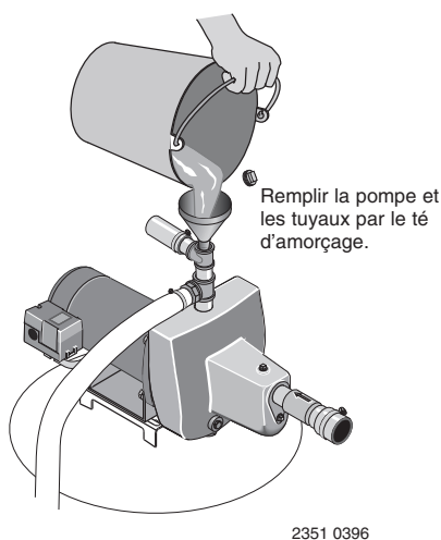
Figure 10 : Amorçage de la pompe
