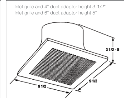
WhisperLine Dimensions
