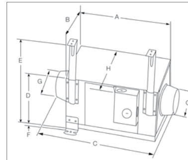
WhisperLine Dimensions
