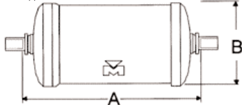
Flare Type
