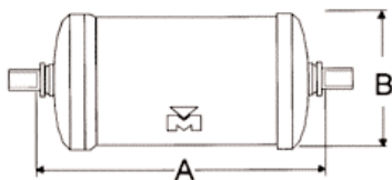
Flare Type
