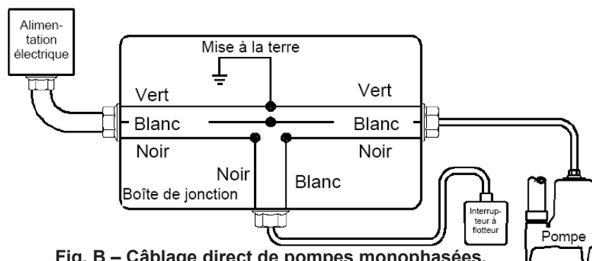
Fig. B – Câblage direct de pompes monophasées, automatiques 120 V ou 208-230 V.
