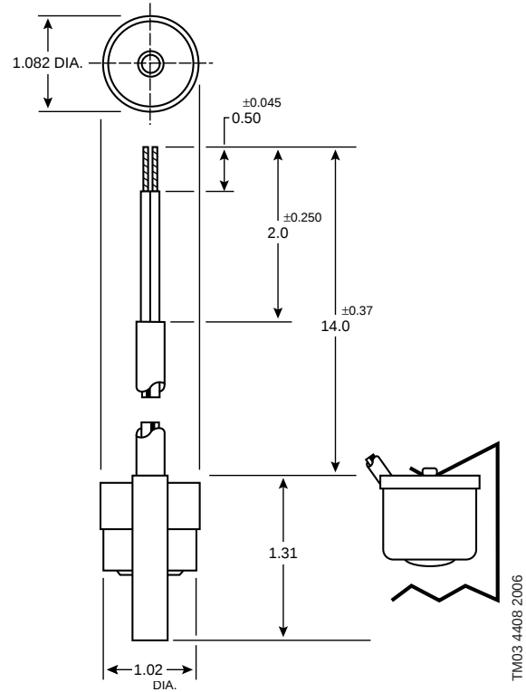
Fig. 13 AquaStat dimensions
