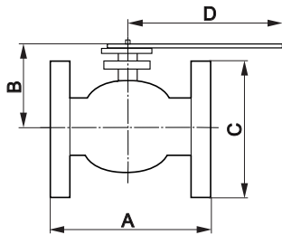
Fig. 16 Dimensions
