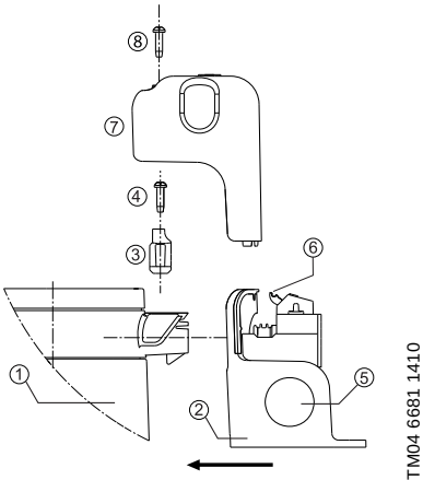
Fig. 3 Installation de la boîte de connexion
