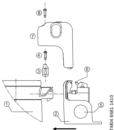
Fig. 3 Instalación de la caja de terminales
