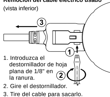
Fig. 1 Remoción del cable eléctrico usado
