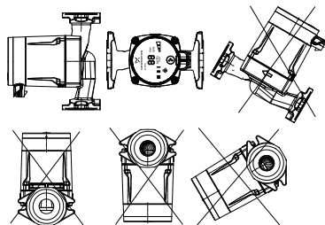
Fig. 2 Positions d'installation
