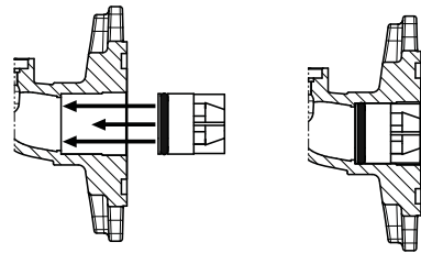
Fig. 1 Verifique la instalación de la válvula
