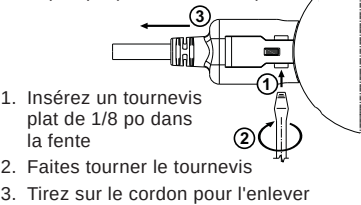
Fig. 4 Branchement et débranchement de la fiche pour les modèles à cordon d'alimentation
