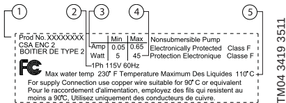
Fig. 6 Plaque signalétique
