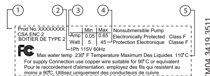
Fig. 6 Placa de identificación del producto
