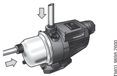
Fig. 4 Fixation des raccords filetés dans les orifices d'aspiration et de refoulement
