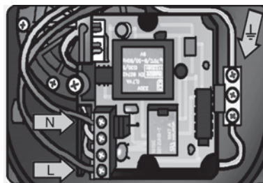
Fig. 10 Conexión eléctrica
