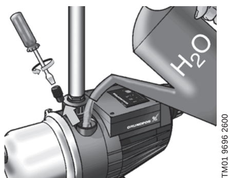
Fig. 14 Amorçage de la pompe
