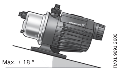
Fig. 2 Instalación horizontal de la bomba MQ
