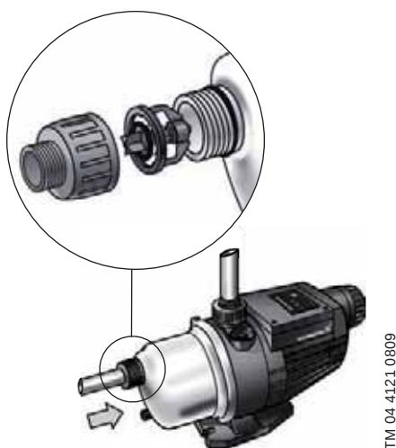
Fig. 8 Installation du clapet d'entrée anti-retour
