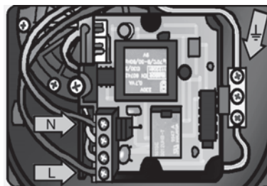
Fig. 10 Branchement électrique
