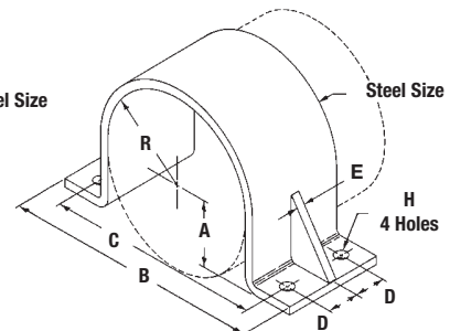
B3256-10 thru B3256-30
